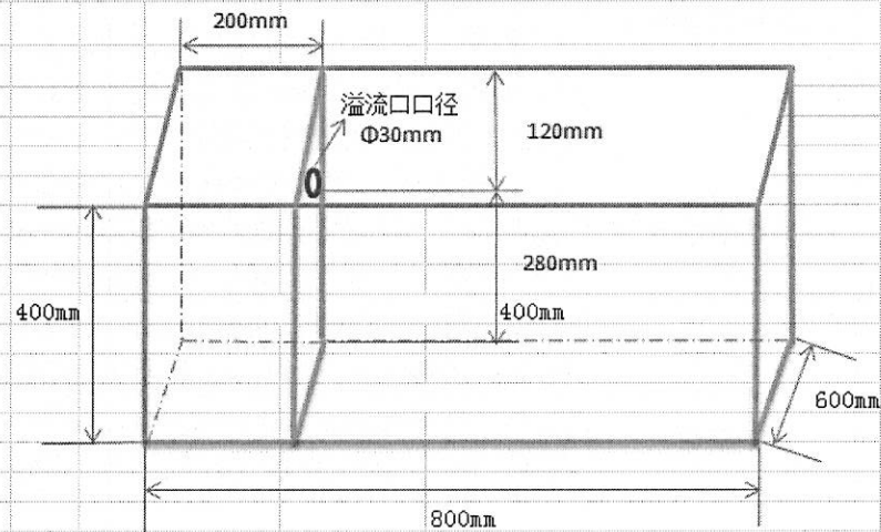
原糖化验室全钢中央实验台两头大水池需分格并且开溢流口，如下图
